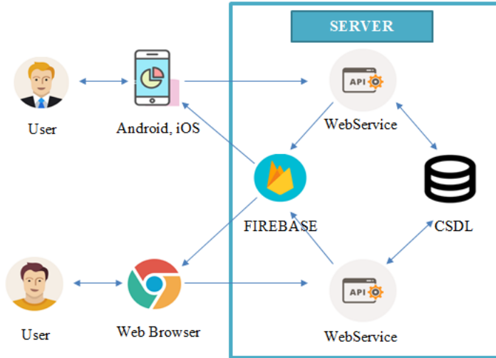
Hình 2: Mô hình tổng thể hệ thống
